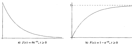
图 8.4 指数分布
