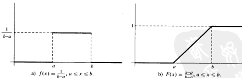
图 8.2 均匀分布
